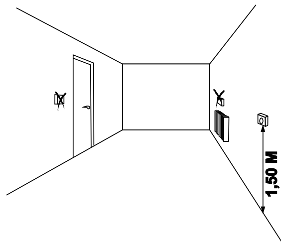
Рисунок 23. Размещение термостатов в помещении
