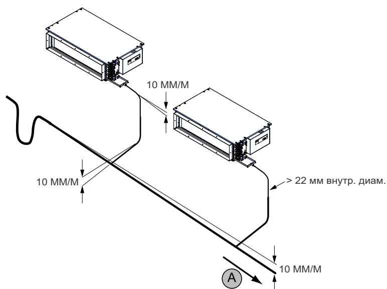
Рисунок 18. Слив из нескольких агрегатов
