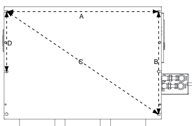
Рисунок 7. Расположение отверстий
