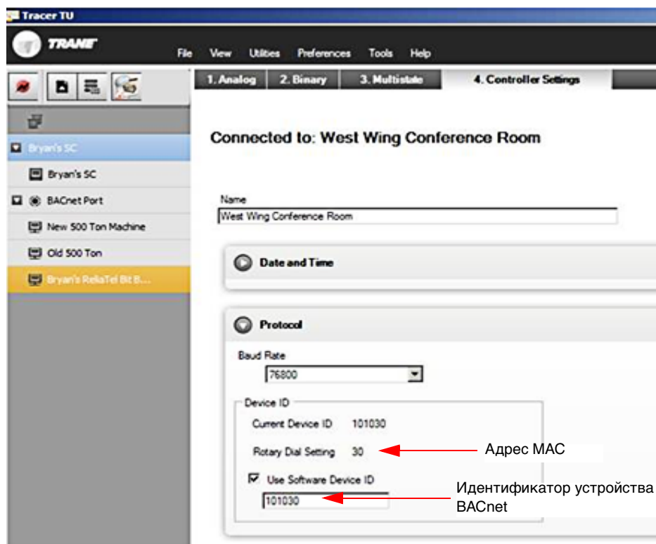
Рисунок 3. Пример установок дискового набора и идентификатора устройства BACnet
