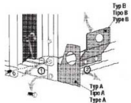
Рисунок 10 - Монтаж ножек основания.
